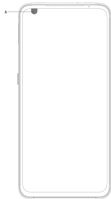
设计3主视图
